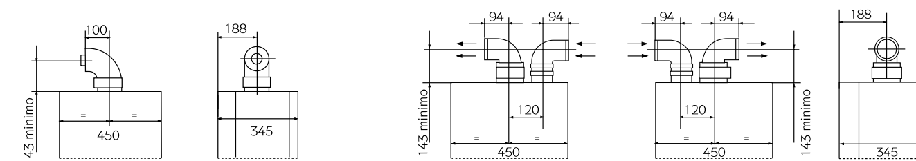
Kit collegamento caldaia/bollitore - KHG714096310
